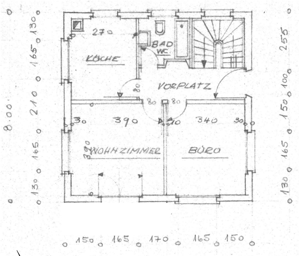
Erdgeschoss
