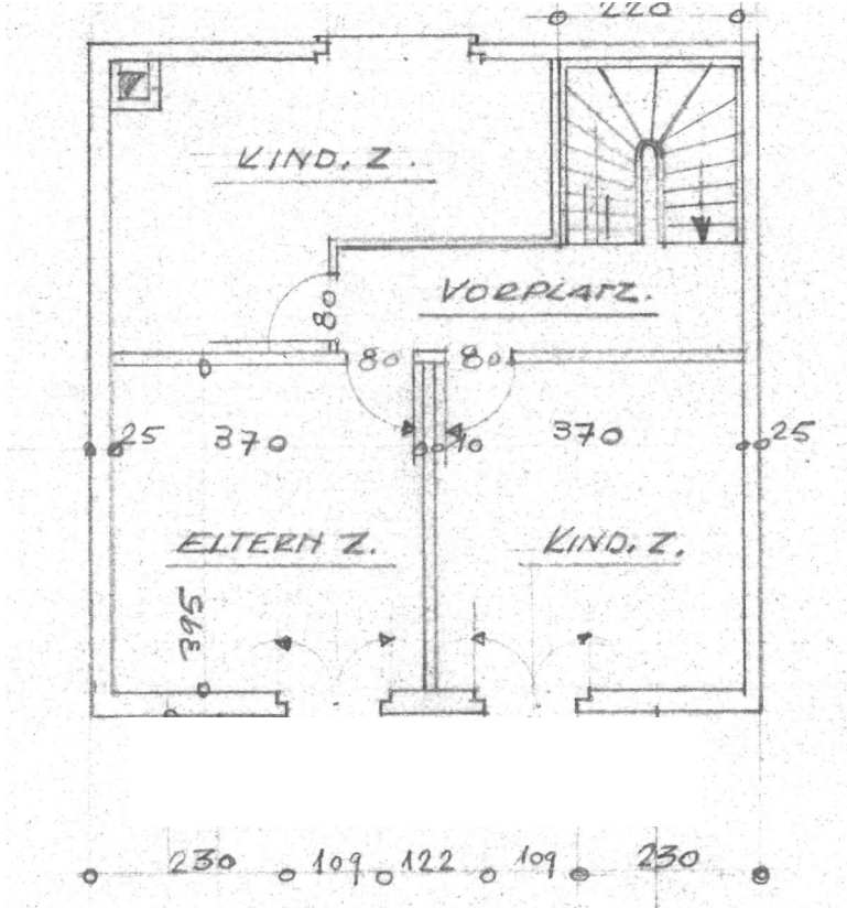
Obergeschoss
