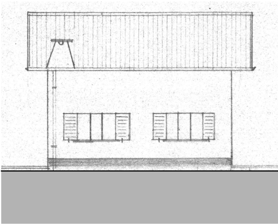
Ansicht West
