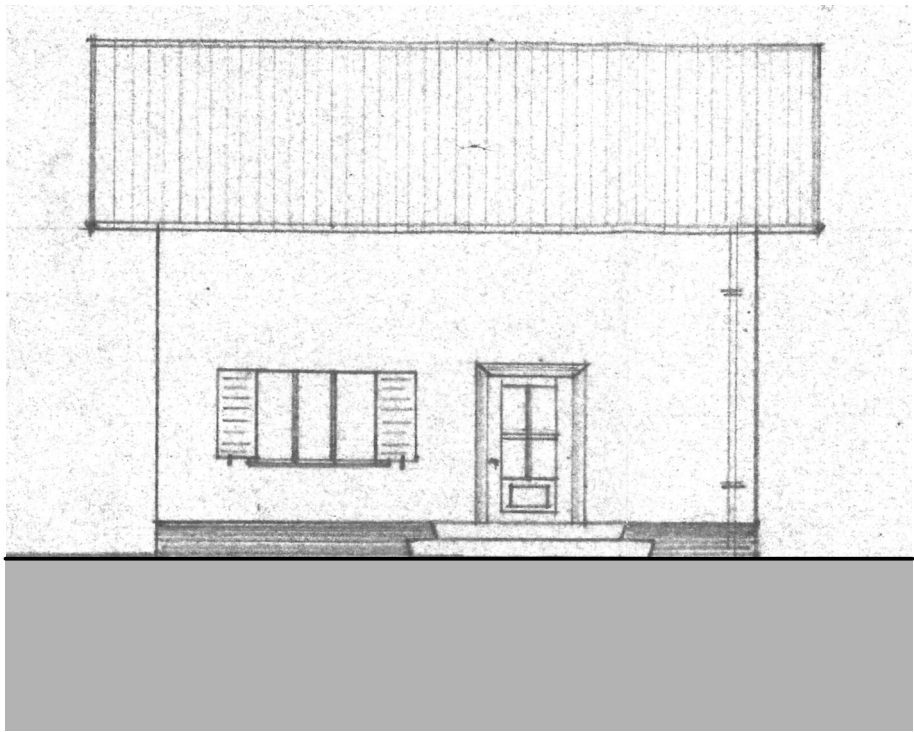
Ansicht Ost
