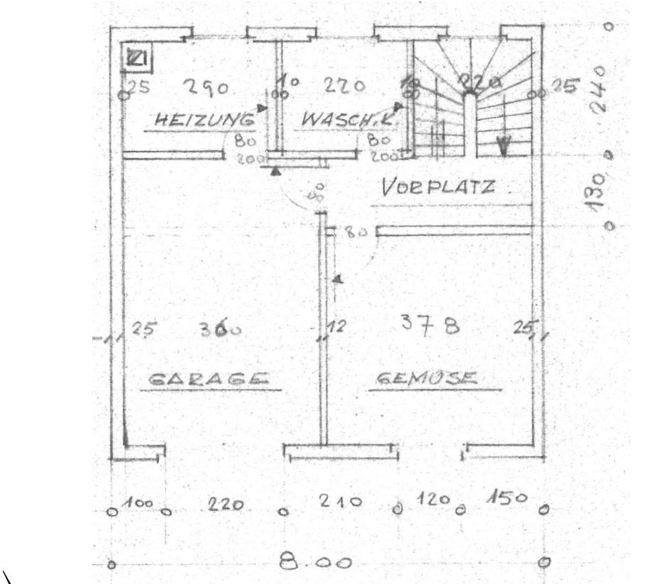
Untergeschoss
