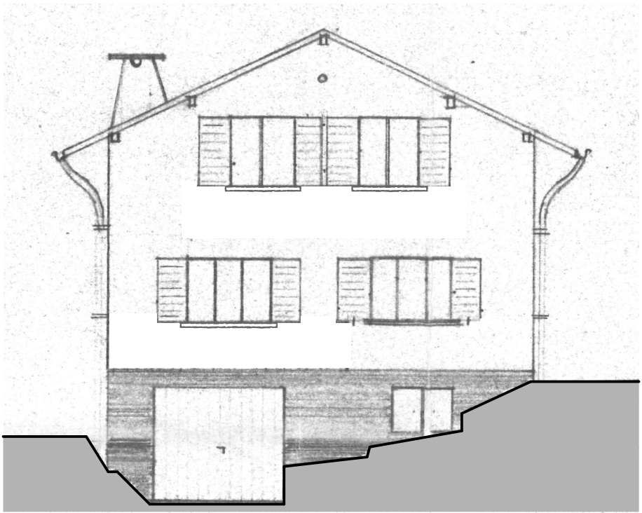
Ansicht Süd
